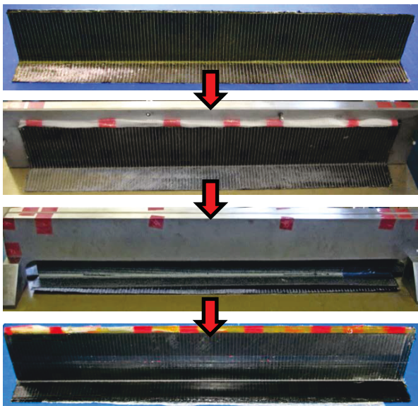
BILD 22. Stringerfertigung: von oben nach unten: Preform alleine; Preform in Werkzeug integriert; geschlossenes Werkzeug mit Druckblechen aus CF-PEEK; entformter Stringer
