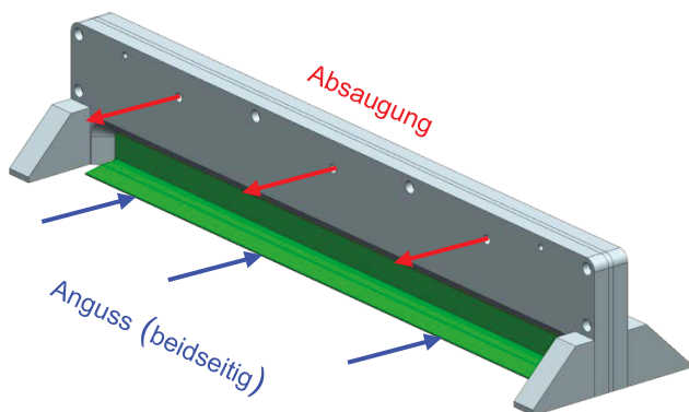
BILD 21. Werkzeug für die Infiltration der Stringer
