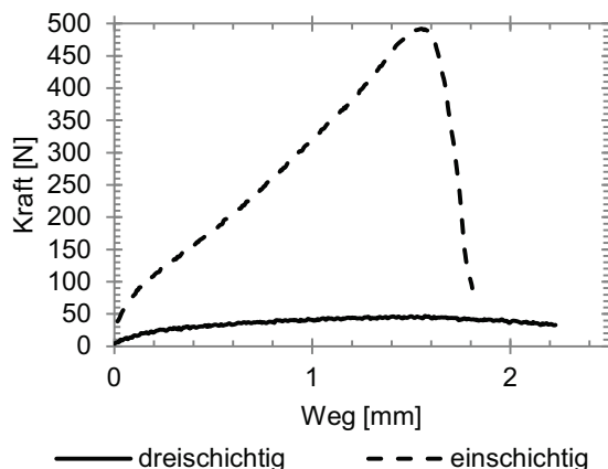
BILD 29. Messwerte von Single-Lap-Shear-Proben
