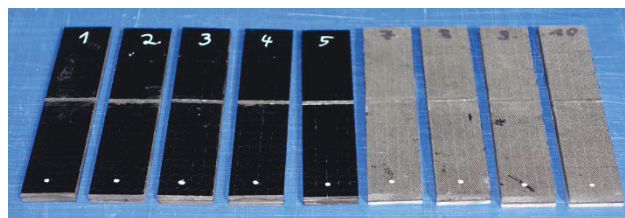
BILD 28. Single-Lap-Shear-Proben
