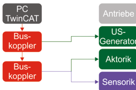
BILD 13. Steuerungskonzept bei Inbetriebnahme außerhalb der Roboterzelle
