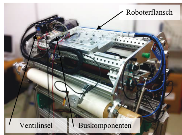
BILD 11. Aufgebauter Endeffektor
